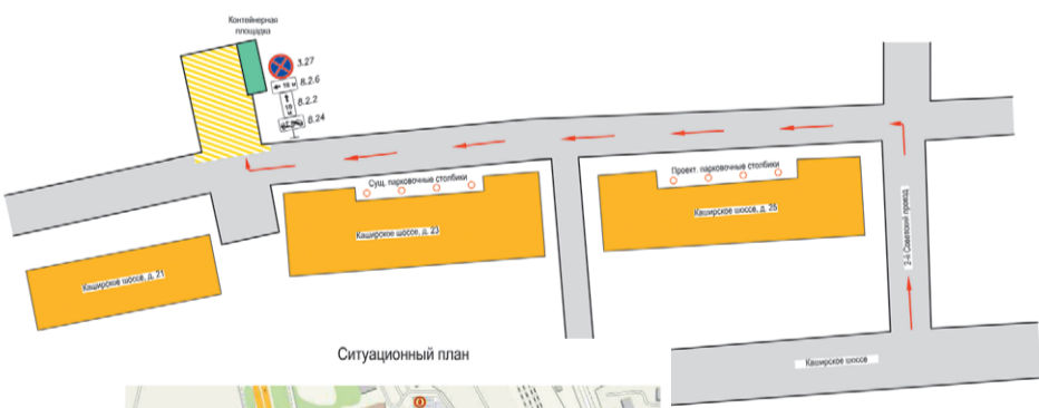
Схема организации дорожного движения по адресу: Московская область, г.о. Домодедово, Каширское шоссе, д. 21, д. 23, д. 25
